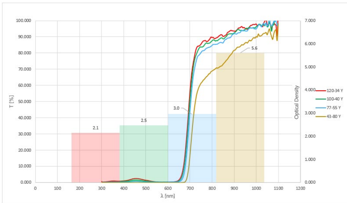
Abbildung 1 Erreichte Deckkraft und IR-Transparenz mit verschiedenen Siebgeweben (Klarlack + Colorant 70:30 mit 3 % Serie 600-HVA) Der Auftrag mit einem Gewebe 43.80 Y ist aufgrund der reduzierten IR-Transparenz nicht für alle Sensoren geeignet, kann aber gegebenenfalls für Spezialanwendungen (z. B. Härtung eines IR-empfindlichen Klebers durch die Farbschicht) interessant sein.
